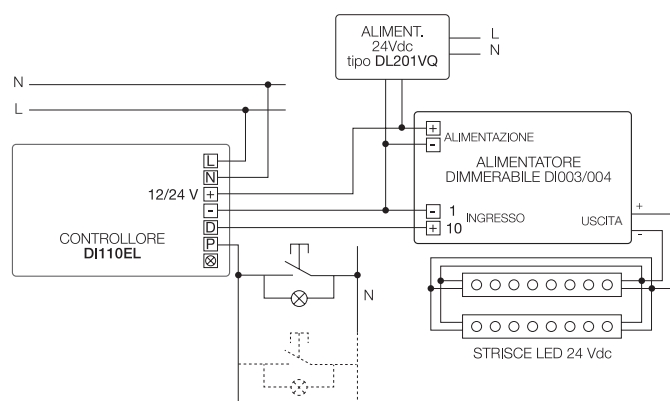
2 Funzionamento con strisce LED 24 V
