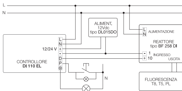
fig. 2 Funzionamento con lampade fluorescenti e carico 230 V dimmerabile
