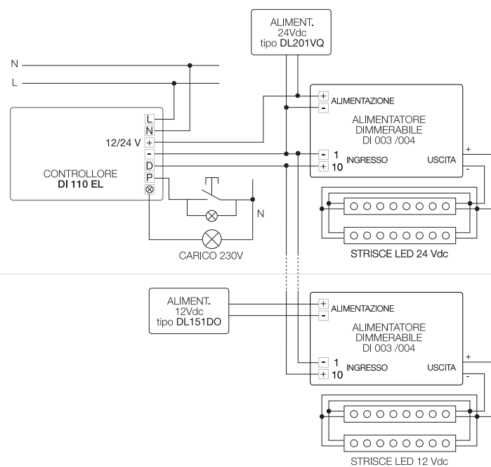
fig. 5 Funzionamento in contemporanea strisce LED 12 V, 24 V e carico 230 V dimmerabile
