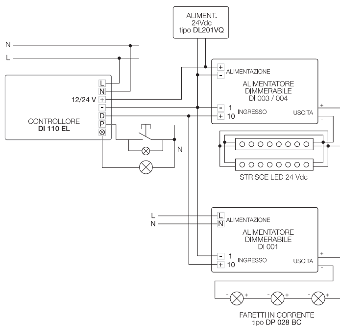
fig. 4 Funzionamento con faretti LED alimentati in corrente costante collegati in serie e carico 230 V
