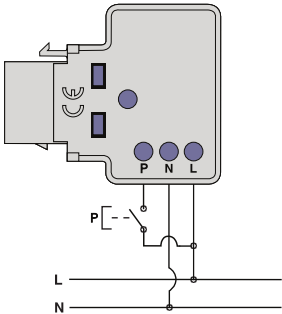
SCHEMA DI COLLEGAMENTO
